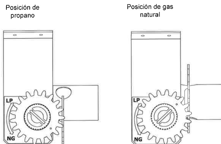
Fig. 8: válvula selectora
