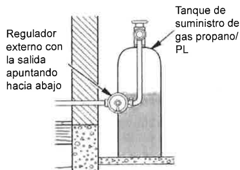
Fig. 9: conversión del regulador
