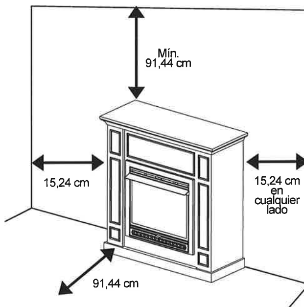
Fig. 6: distancia de separación mínima con materiales combustibles
