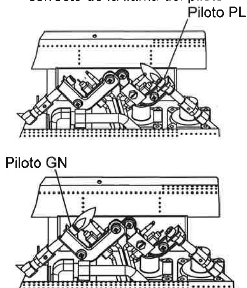
Fig. 20: comportamiento correcto de la llama del piloto
