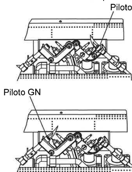
Fig. 21: comportamiento incorrecto de la llama del piloto
