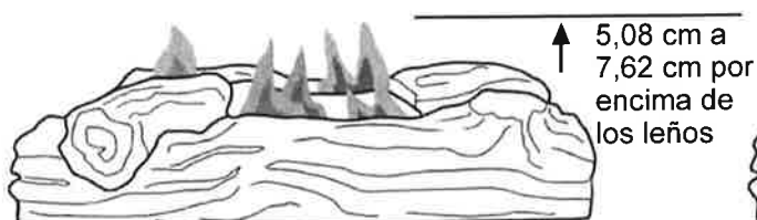
Fig. 22: comportamiento correcto de la llama del quemador
