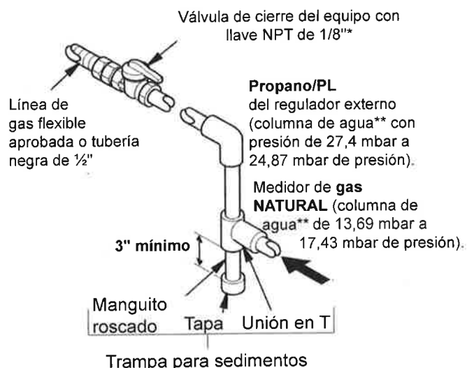
Fig. 10: conexión de gas
